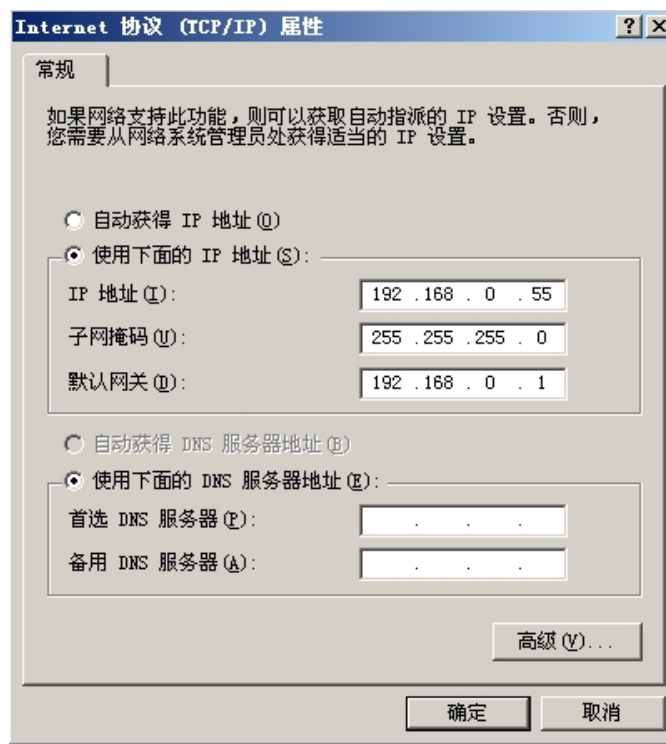
图 4-7. Internet 协议(TCP/IP)属性
