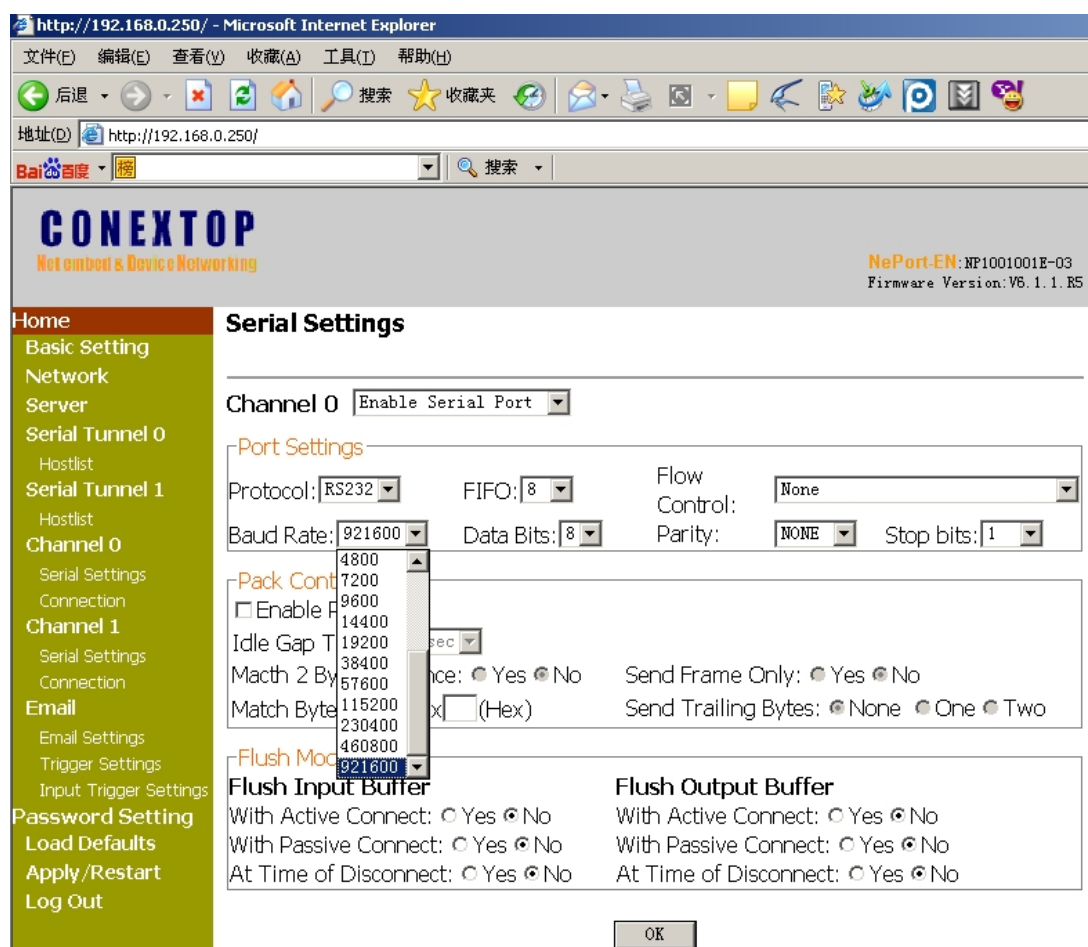
图 5-4. 串口配置页面
