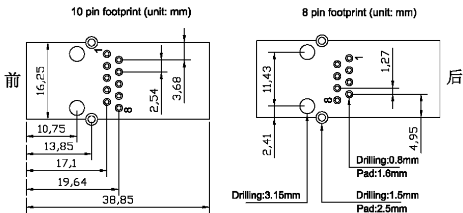
图2-7. 推荐的PCB封装
