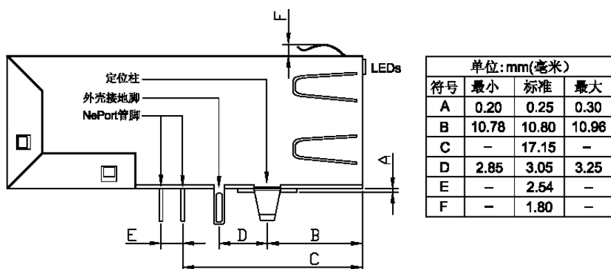
图2-6. 侧面图
