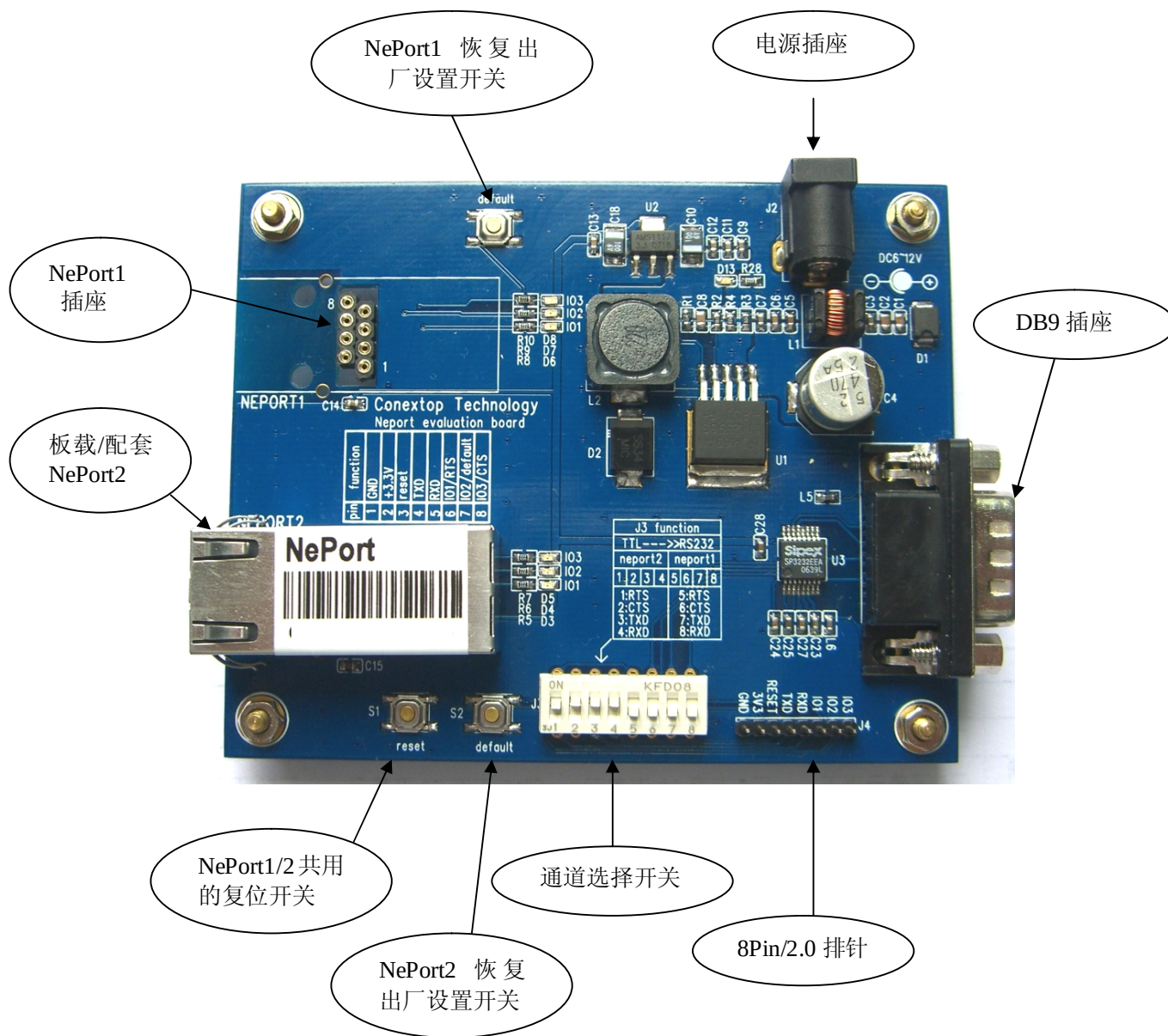
图 2-11. 评估板
