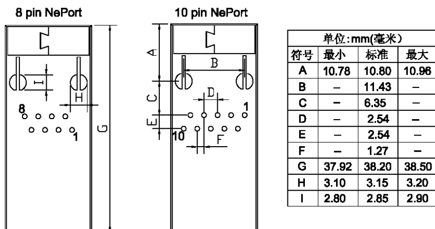
图2-6. 侧面图
