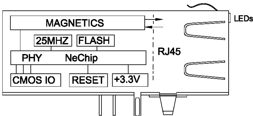
图2-1. 侧面剖析图
