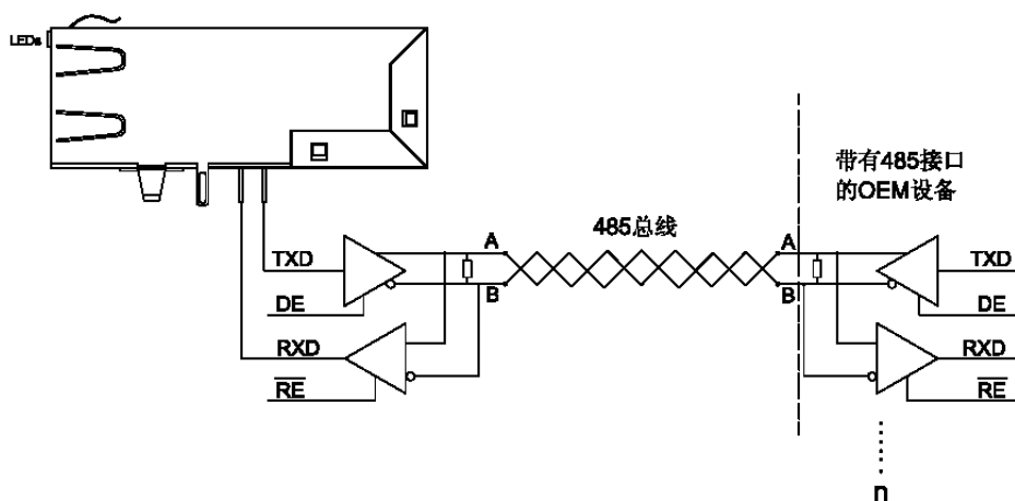
图 3-2. RS422 连接示意图
