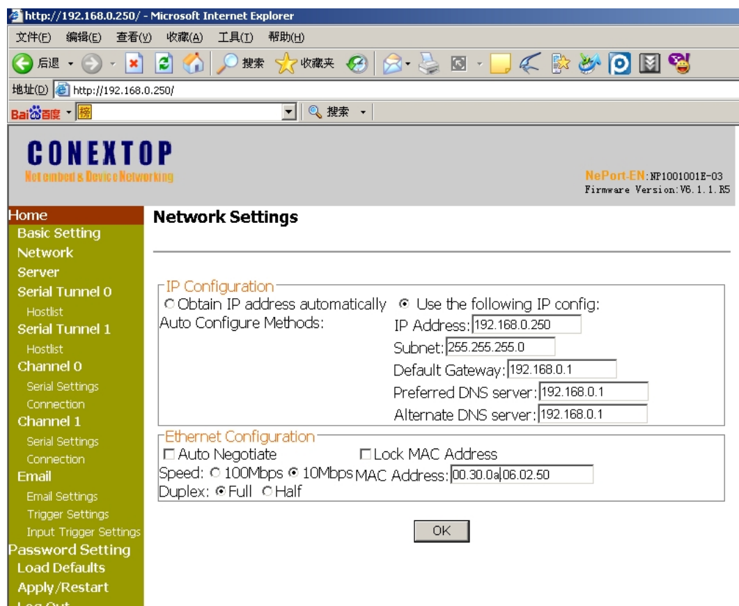
图 5-3. 网络配置
