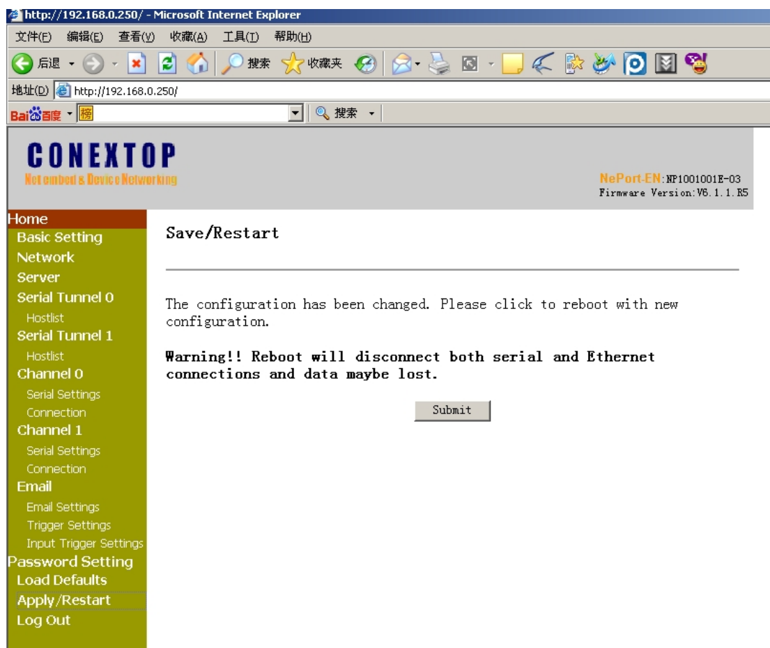
图 5-8. Apply/Restart 页面
