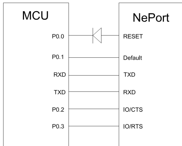
图2-8. 推荐的复位联接方式
