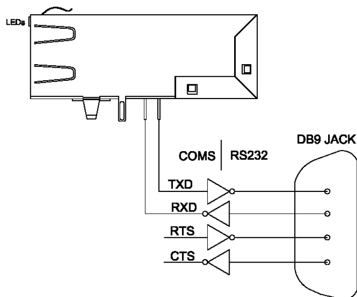
图 3-3. RS232 连接示意图
