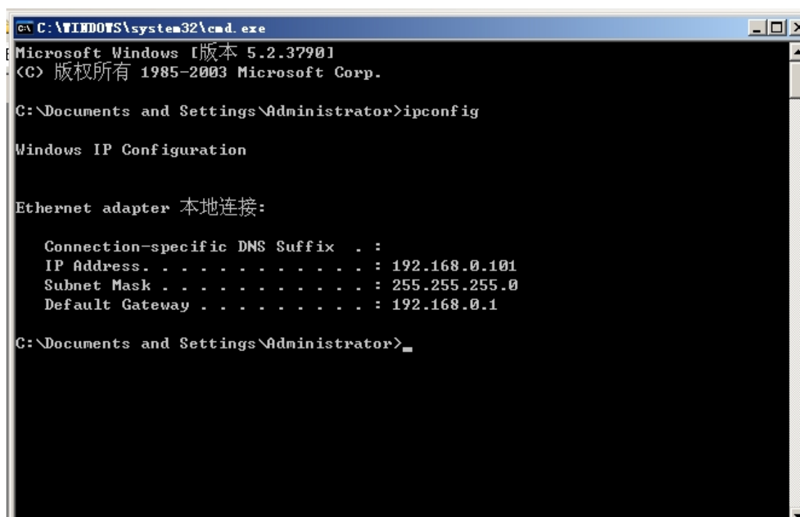
图 4-1. cmd.exe 窗口
