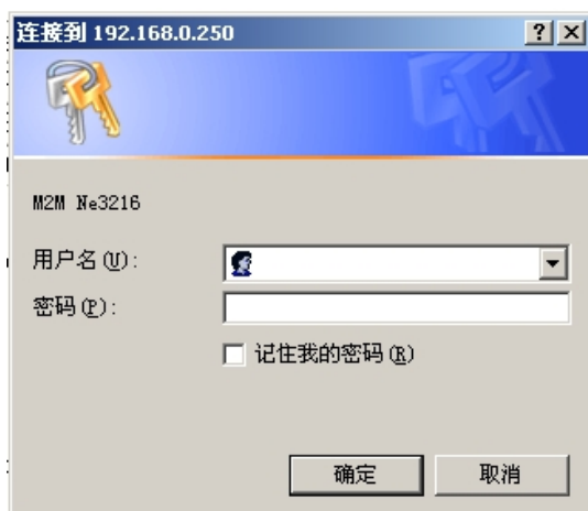
图 5-1. 登入窗口
