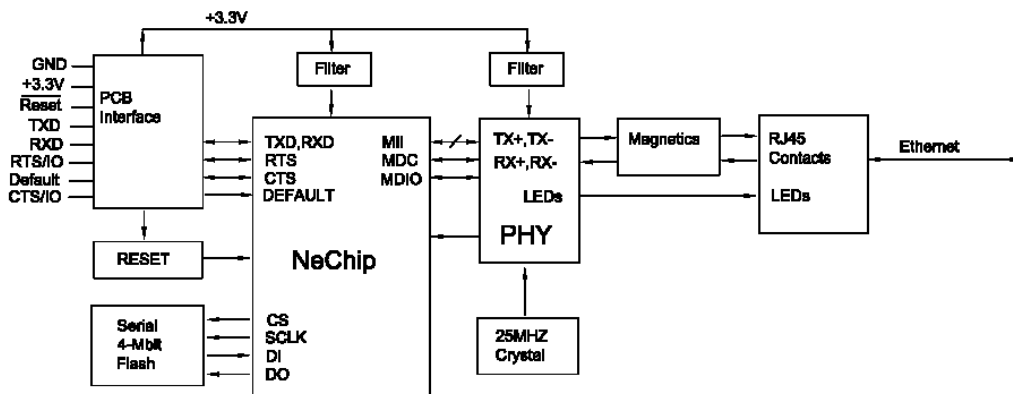
图2-2. 方框图
